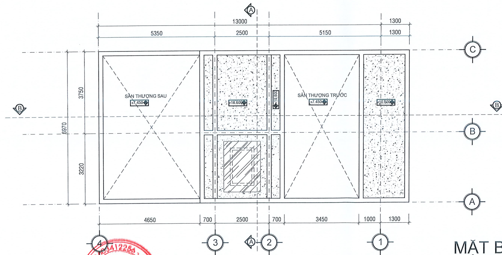
MẶT BẰNG TẦNG TUM TL: 1/100
