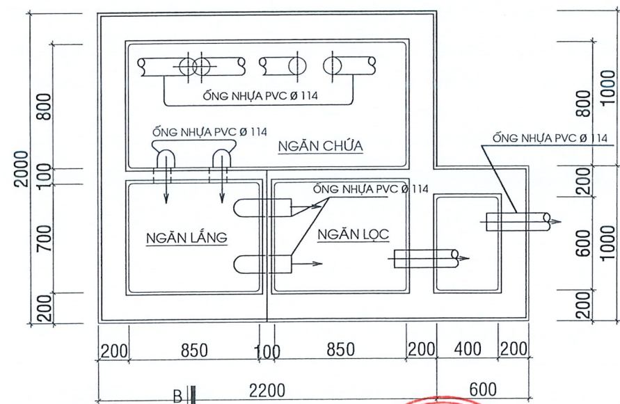
MB HẠM TỰ HOẠI TL: 1/25
