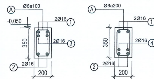
Gối Nhịp DK1 (200X350) TL 1:25
