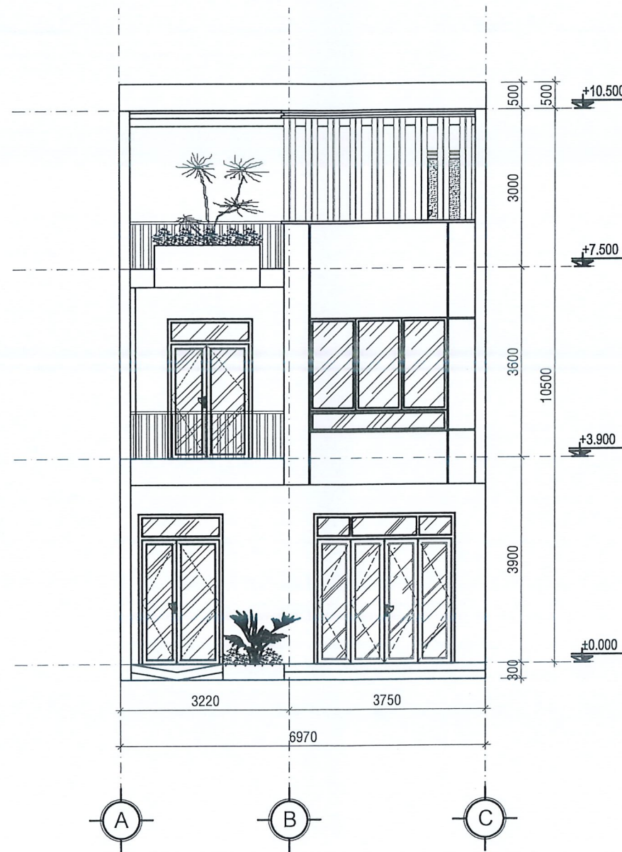
MẶT ĐƯỜNG A-C TL: 1/100
