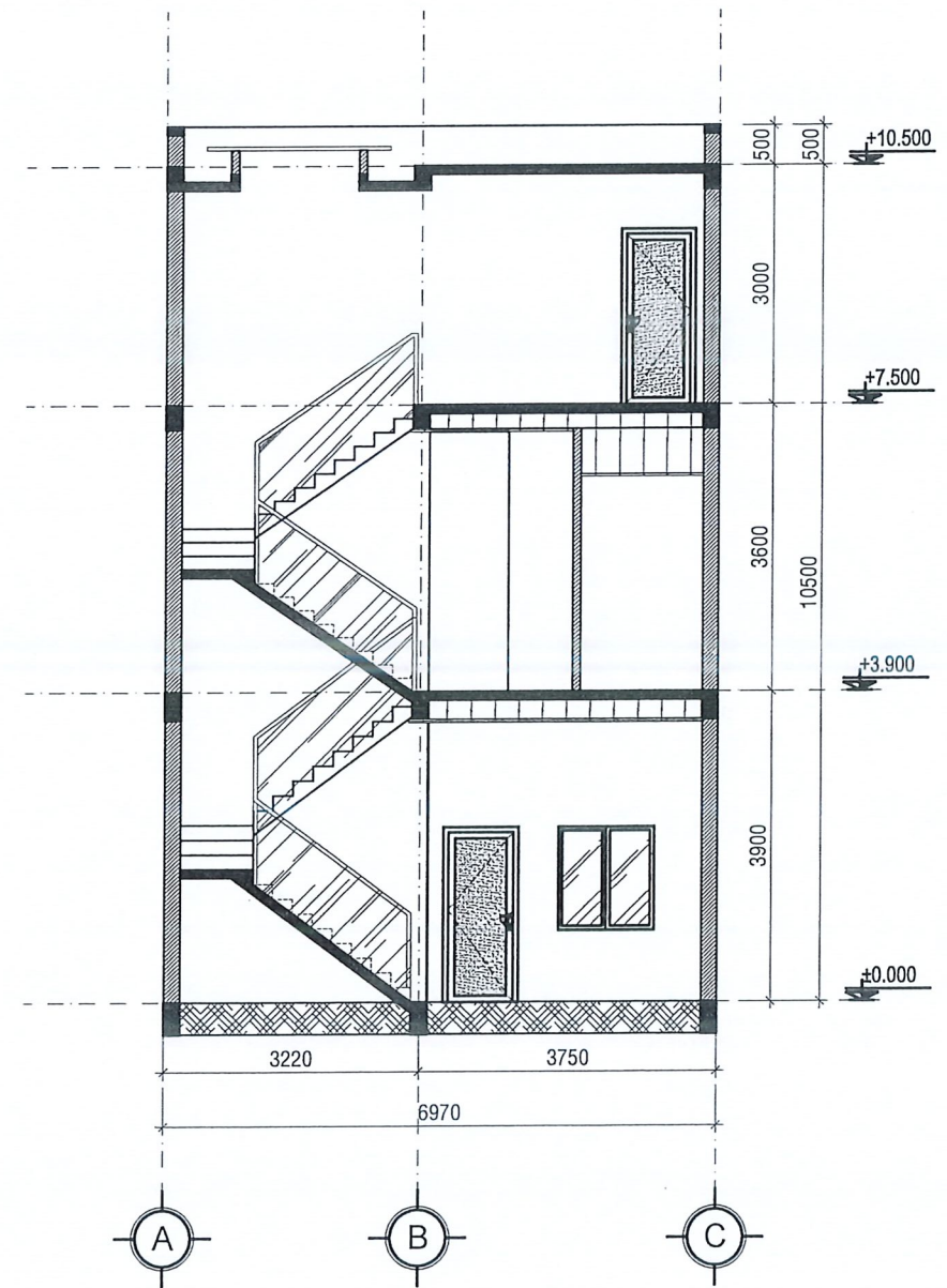
MẶT CẮT A-A TL: 1/100
