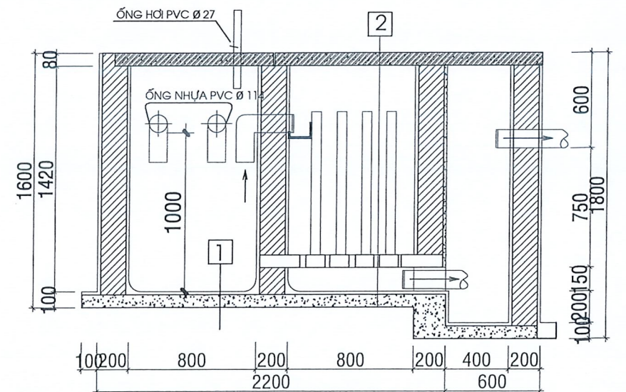
MC B-B TL: 1/25
