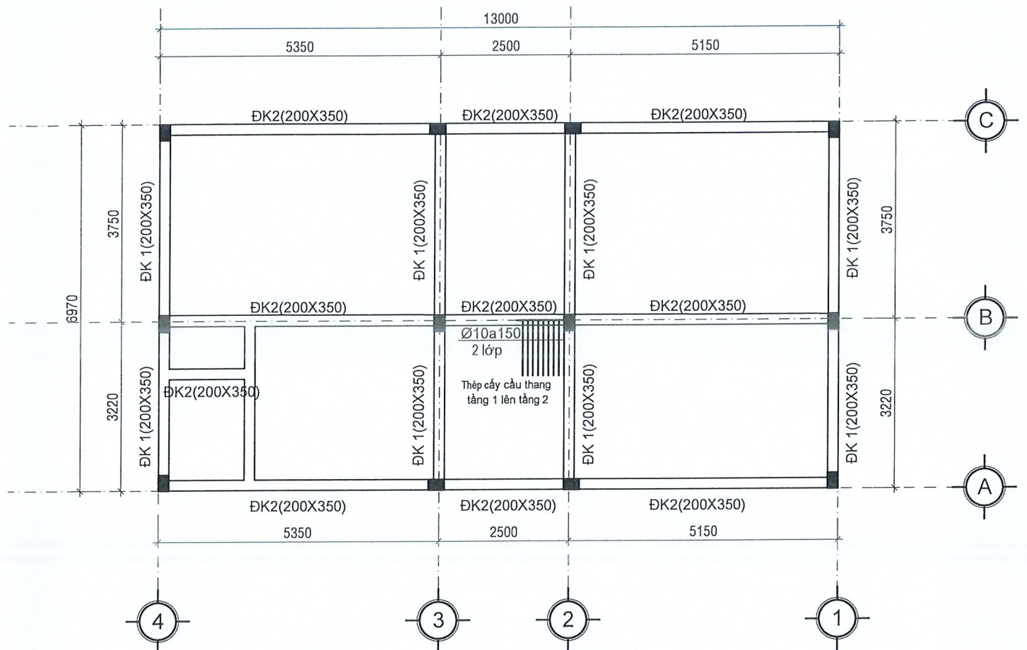
MẶT BẰNG BỐ TRÍ ĐÀ KIỀNG TL: 1/100
