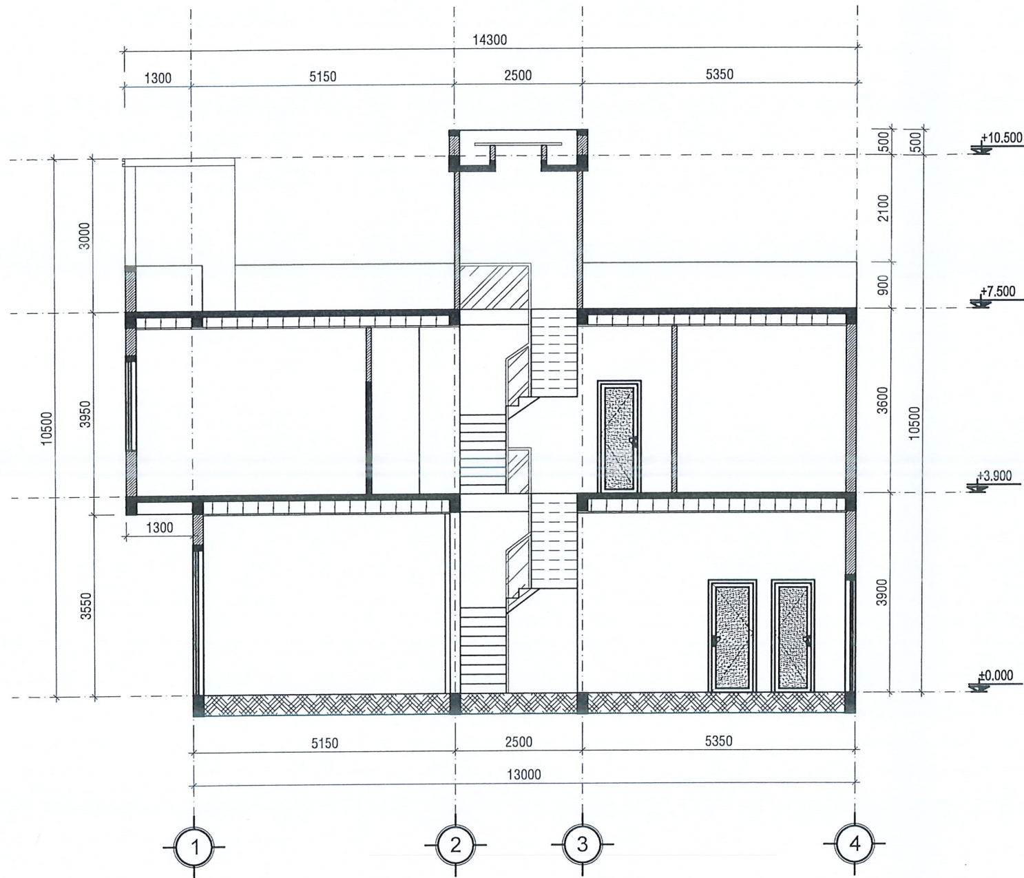
MẶT CẮT B-B TL: 1/100
