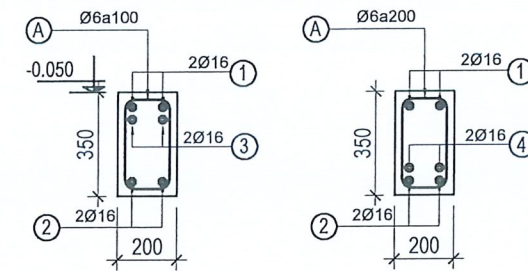
Gối Nhịp DK2 (200X350) TL 1:25
