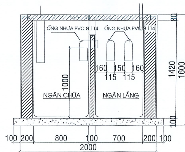
MC B-B TL: 1/25
