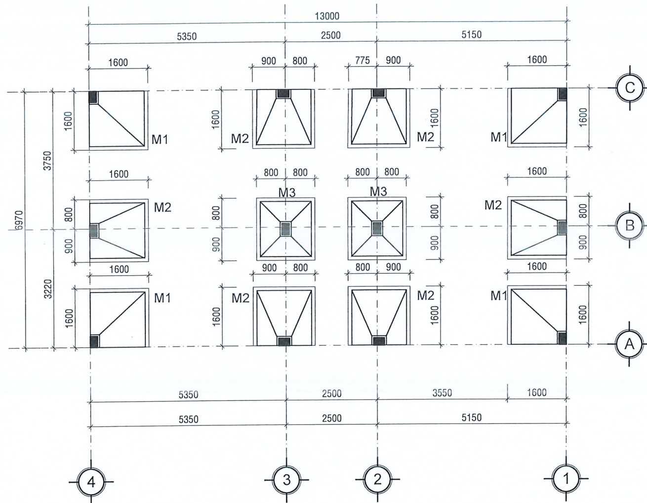
MẶT BẰNG BỐ TRÍ MÓNG TL: 1/100
