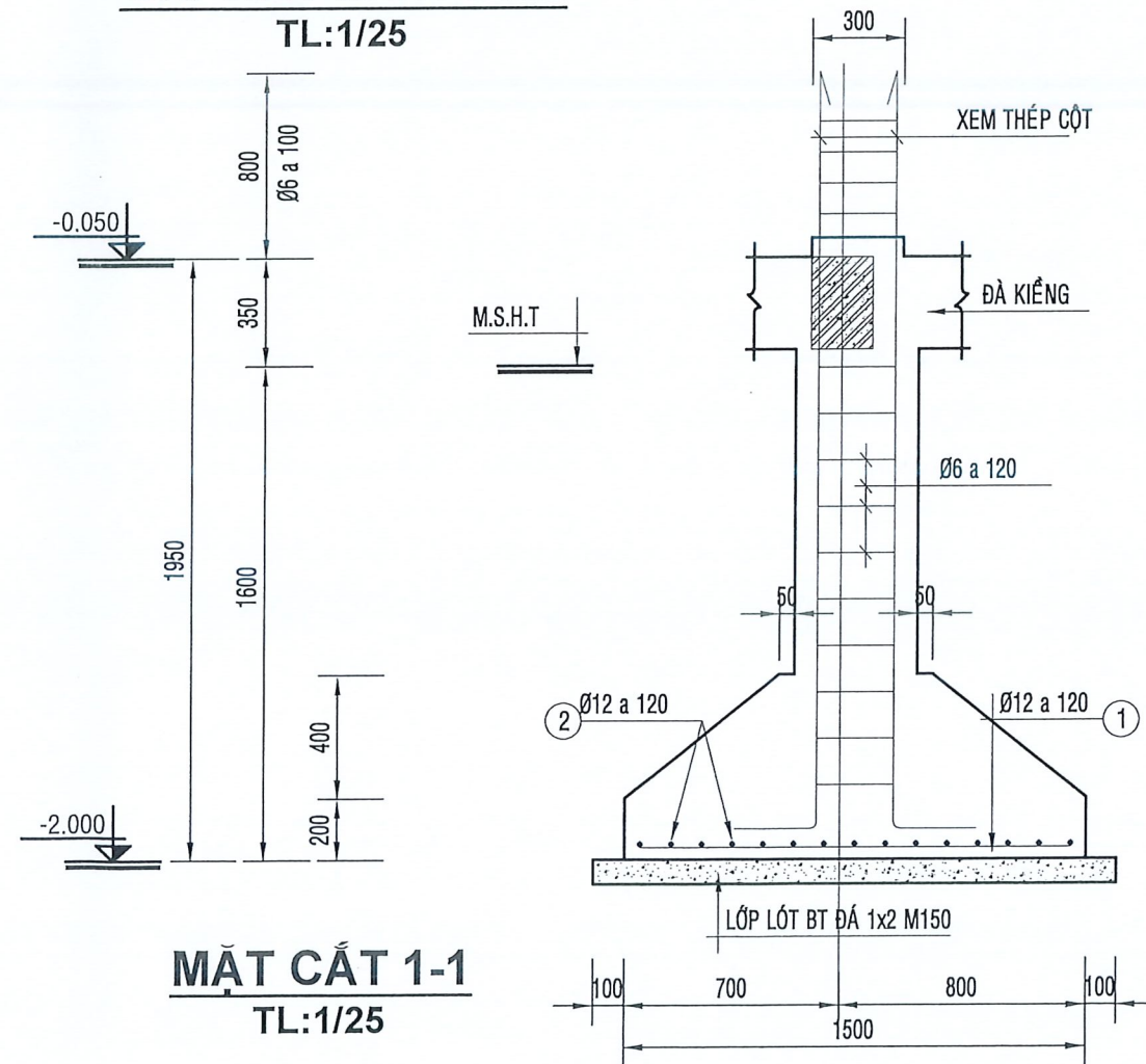
CHI TIẾT MÓNG M2
