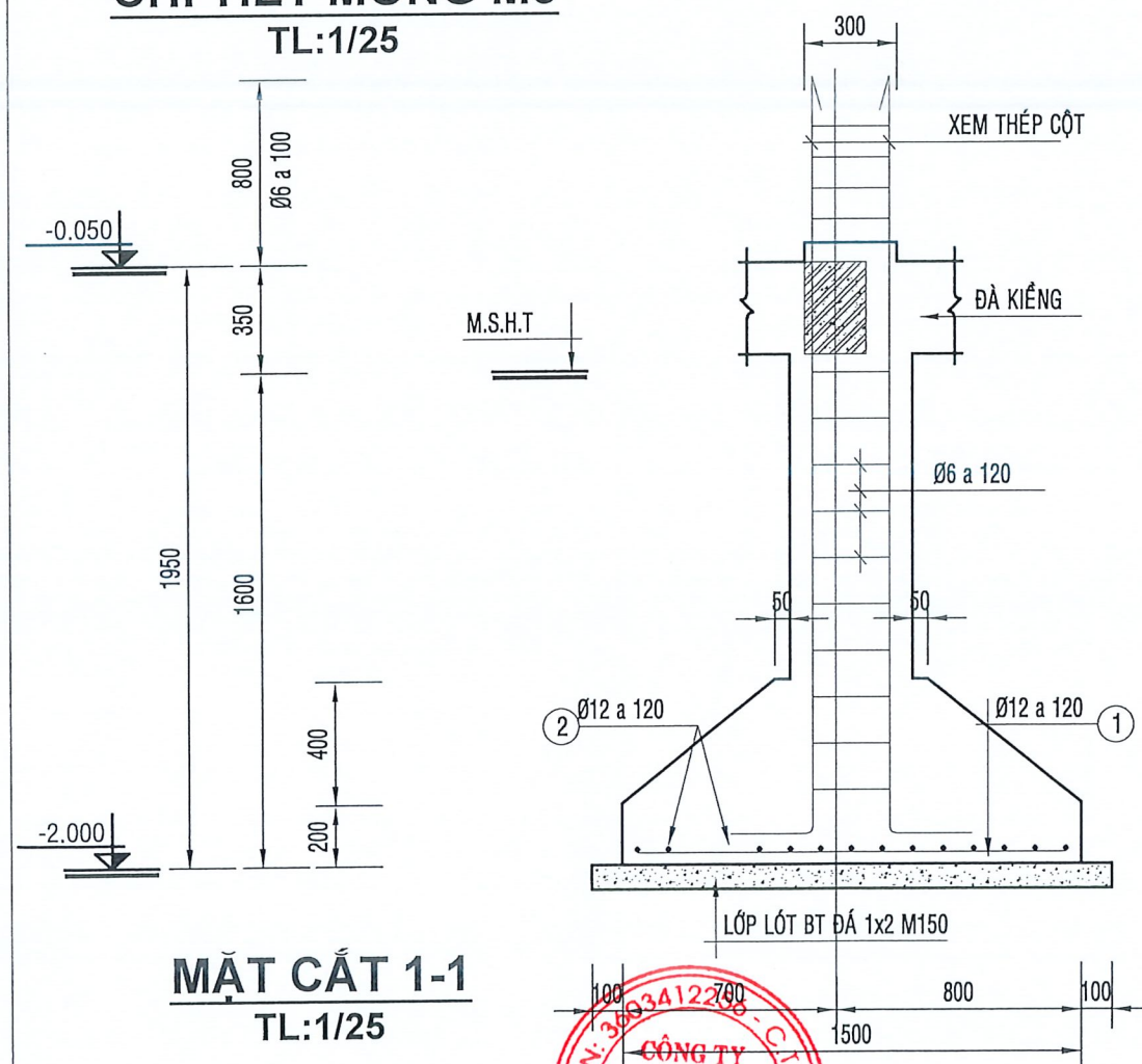
CHI TIẾT MÓNG M3
