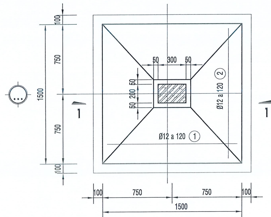
CHI TIẾT MÓNG M3
