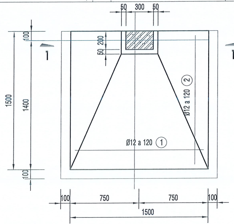
CHI TIẾT MÓNG M2
